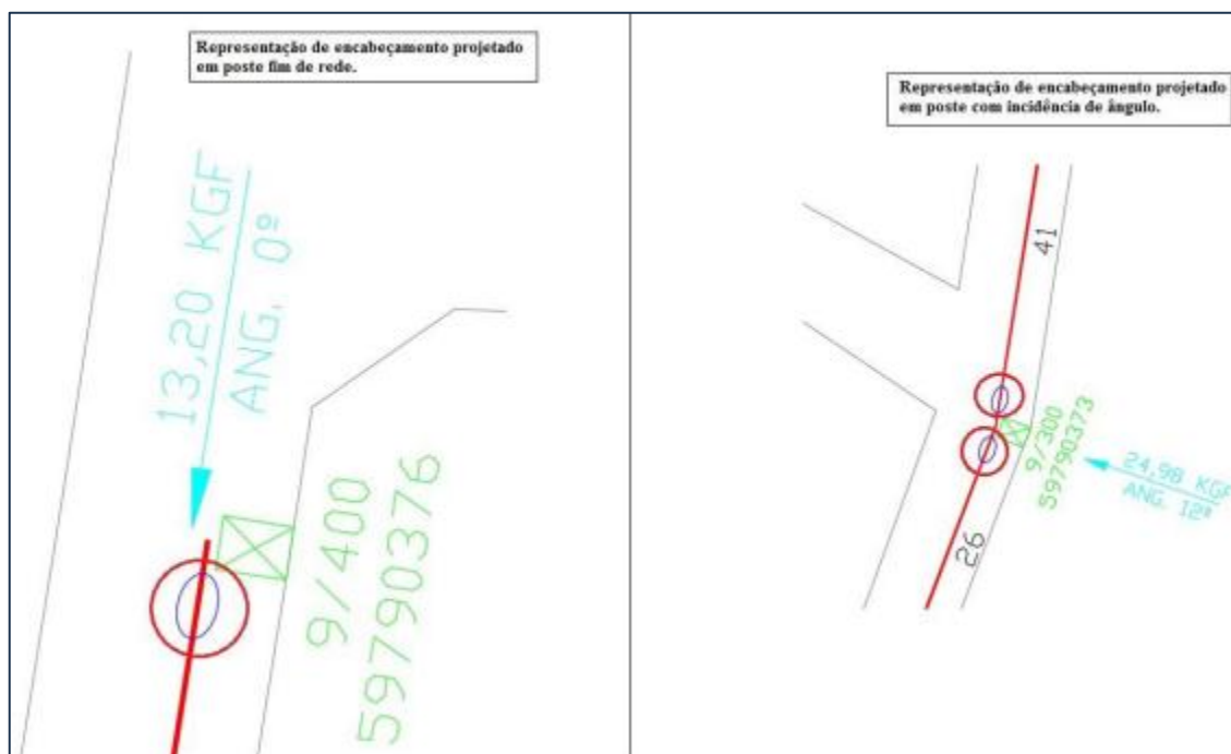
Figura 10. Representação de simbologia de encabementos projetados.
