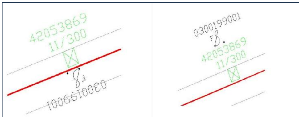
Figura 02. Representação correta de equipamento especial em poste.
