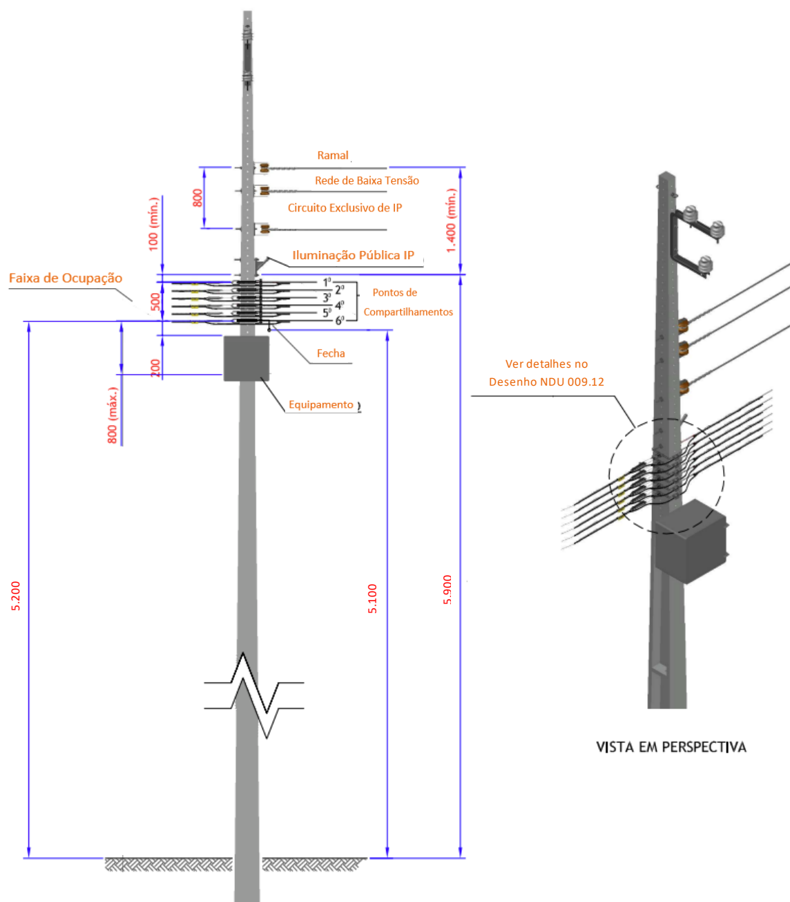
Rede Padrão Compacto (Spacer Cable)
