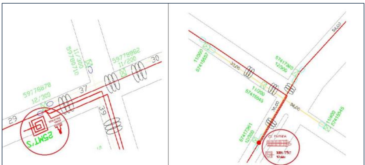
Figura 07. Representação de Caixas de Emendas.
